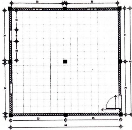
⊙ DENAH PEMASANGAN KERAMIK 40X40 CM BANGUNAN BARU
