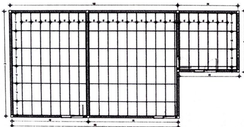
⊙ DENAH PEMASANGAN RANGKA HOLLOW 4X4 CM BANGUNAN BARU
